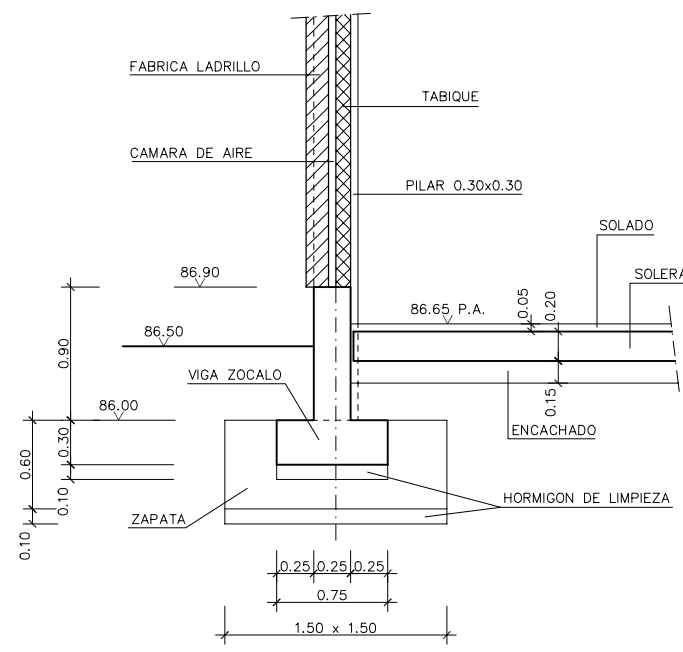
SECCION A-A ESCALA 1:25
