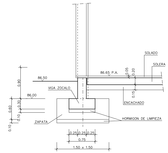
SECCION B-B ESCALA 1:25
