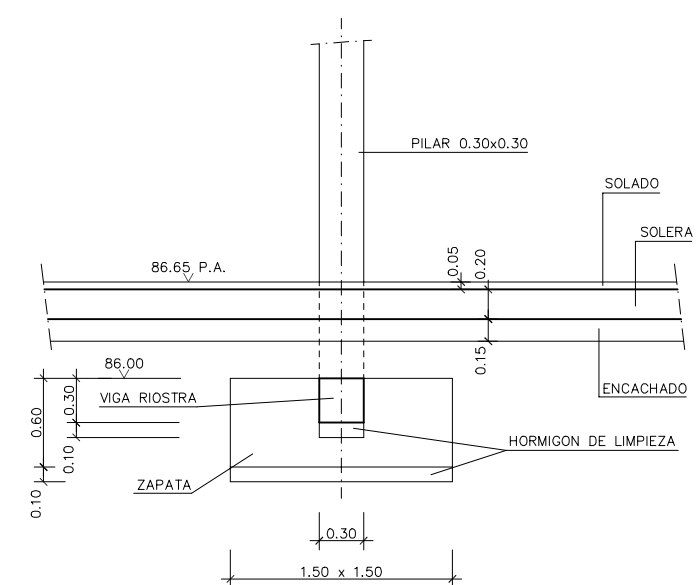
SECCION C-C ESCALA 1:25
