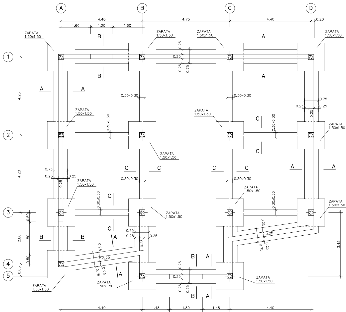
PLANTA BAJA ESCALA 1:50
